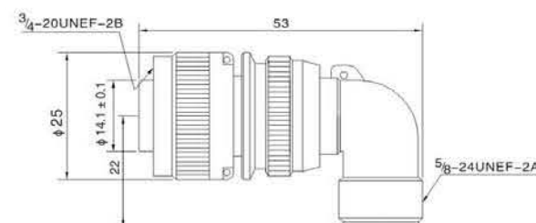
MS3108A 90°弯式插头 MS3108A 90°-angle Plug
