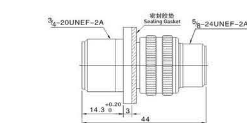
MS3100A 墙式方盘安装插座 MS3100A Wall Mounting Receptacle
