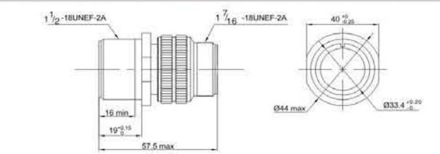
MS3101 中继插座 MS3101 Cable Connecting Socket
