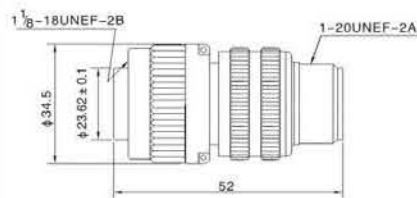
MS3101 中继插座 MS3101 Cable Connecting Socket
