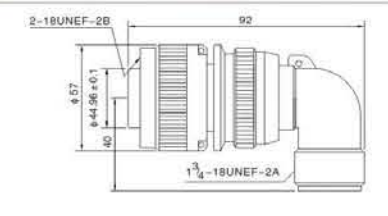
MS3108A 90°弯式插头 MS3108A 90°—angle Plug
