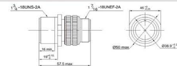
MS3101 中继插座 MS3101 Cable Connecting Socket
