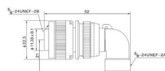
MS3108A 90°弯式插头 MS3108A 90°-angle Plug
