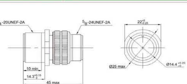
MS3101 中继插座 MS3101 Cable Connecting Socket
