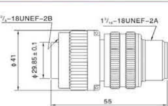
MS3106A 直式插头 MS3106A Straight Plug
