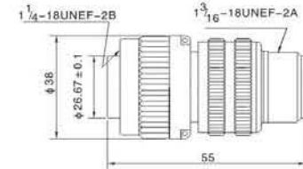
MS3101 中继插座 MS3101 Cable Connecting Socket
