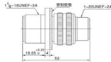
MS3100A 墙式方盘安装插座 MS3100A Wall Mounting Receptacle
