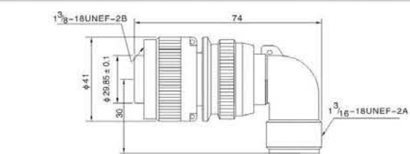
MS3108A 90°弯式插头 MS3108A 90°—angle Plug
