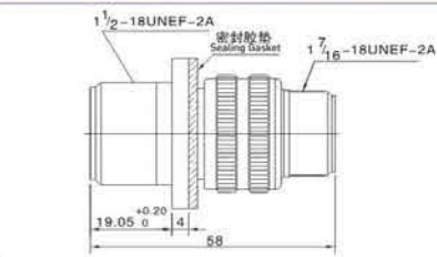
MS3100A 牆式方盤安裝插座 MS3100A Wall Mounting Receptacle
