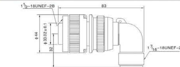
MS3108A 90°弯式插头 MS3108A 90°—angle Plug
