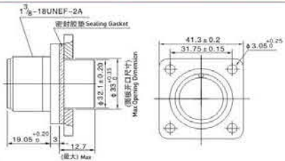
MS3102 盒式方盘安装插座 MS3102 Box Mounting Receptacle
