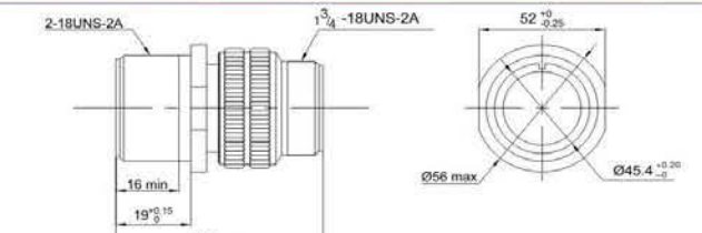
MS3101 中继插座 MS3101 Cable Connecting Socket
