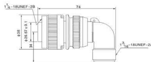
MS3108A 90°弯式插头 MS3108A 90°-angle Plug
