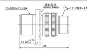
MS3100A 墙式方盘安装插座 MS3100A Wall Mounting Receptacle
