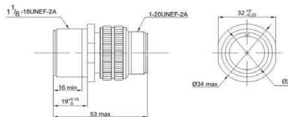
MS3101 中继插座 MS3101 Cable Connecting Socket
