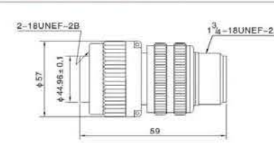
MS3106A 直式插头 MS3106A Straight Plug
