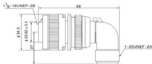
MS3108A 90°弯式插头 MS3108A 90°-angle Plug
