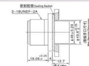
MS3102 盒式方盘安装插座 MS3102 Box Mounting Receptacle
