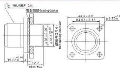
MS3102 盒式方盘安裝插座 MS3102 Box Mounting Receptacle
