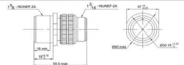
MS3101 中继插座 MS3101 Cable Connecting Receptacle
