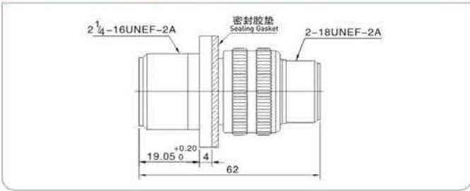
MS3100A 墙式方盘安装插座 MS3100A Wall Mounting Receptacle
