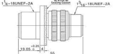
MS3100A 墙式方盘安装插座 MS3100A Wall Mounting Receptacle
