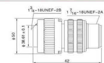
MS3106A 直式插头 MS3106A Straight Plug
