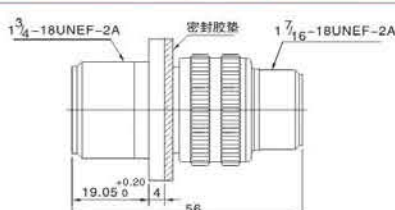
MS3100A 牆式方盤安裝插座 MS3100A Wall Mounting Receptacle
