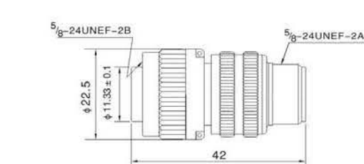
MS3106A 直式插头 MS3106A Straight Plug
